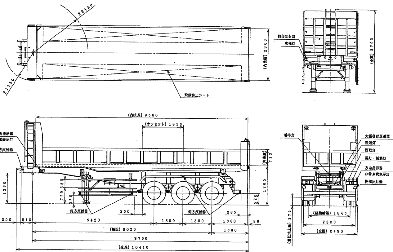
コダイラ KFL32改 ダンプセミトレーラ外觀四面図
